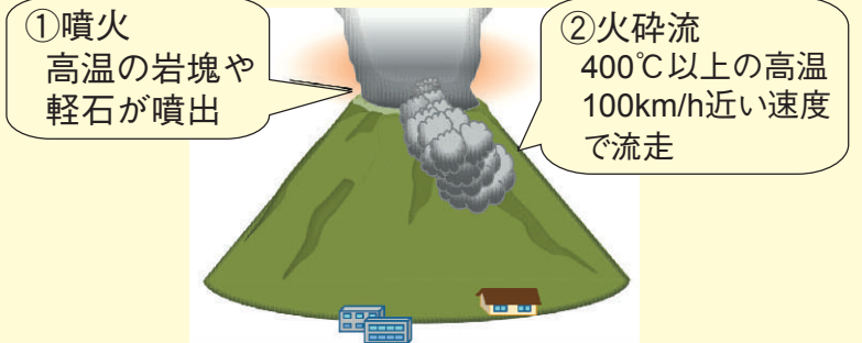
火砕流イメージ図
