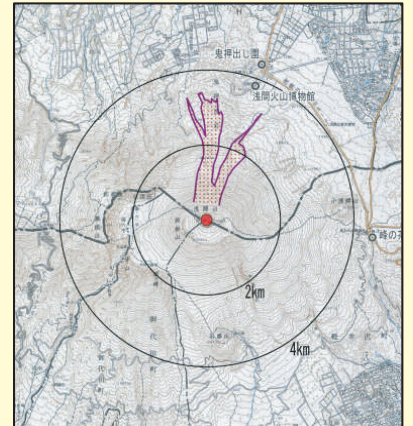
1982年 融雪泥流 火口から約3.5kmに到達
